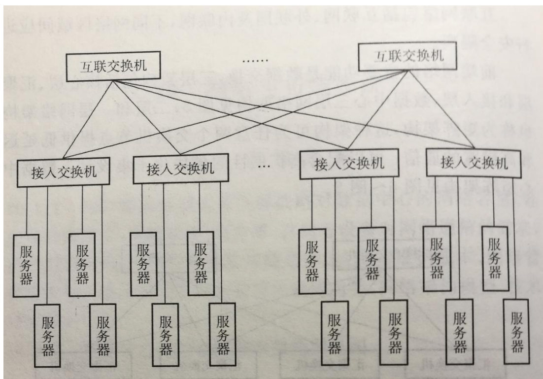
图 6 数据中心矩阵架构图(一)
