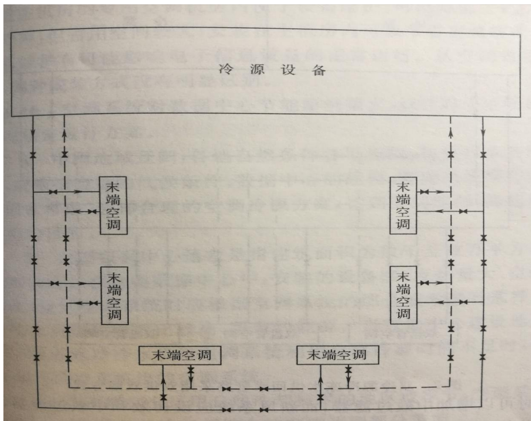
图1 冷冻水供回水管路采用环形管网方式
