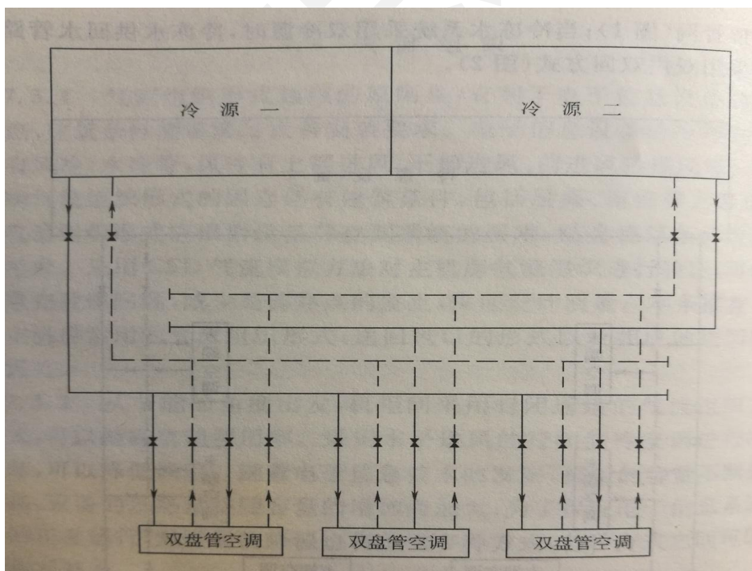
图2 双冷源冷冻水供回水管路采用双供双回方式
